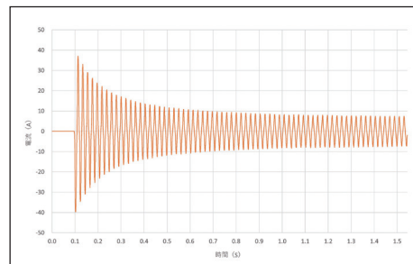
(図4) 突入電流
